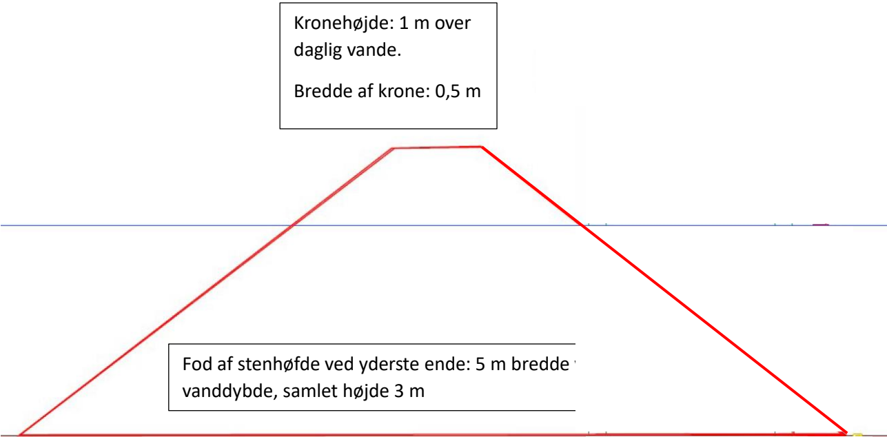
Bilag 2 - Tværsnit for stenhøfder, Østerstrand 2024
