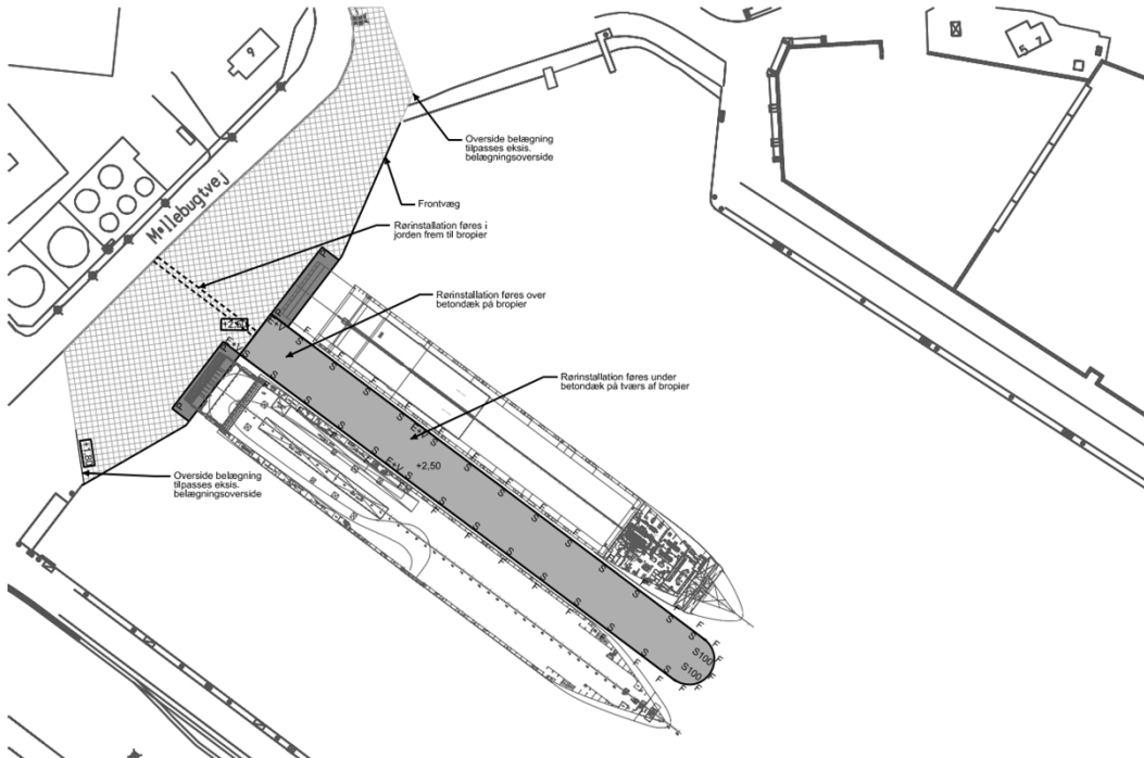
Figur 3-1 i notatet med projektændringer ved kaj 23: Kaj 23 projektet opdateret – én lang bropier.
