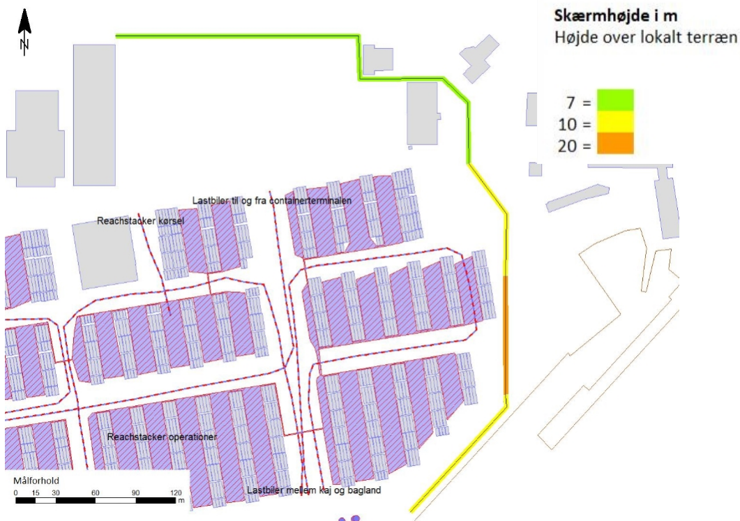
Figur 12-26 fra miljøkonsekvensrapporten: Oversigtskort for fremtidig containerterminal med angivelse af støjskærme og højder.
