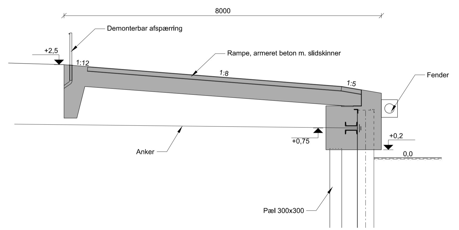
Snit Ro-ro rampe (1:50) (vist som princip)
