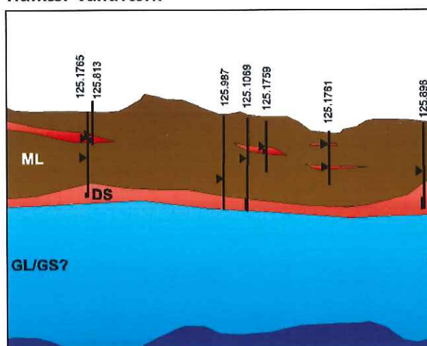
Figur 25: Geologisk principsnit omkring Tiufkær Vandværks kildeplads med angivelse af borerplaceringer (vest-øst), se figur 26. (Legende henvises til figur 21.)
