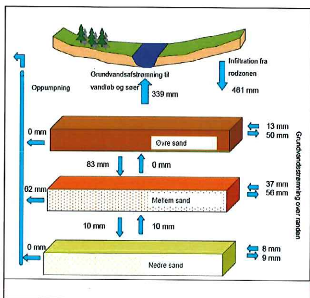
Figur 8. Vandbalance for Follerup Indsatsområde.
