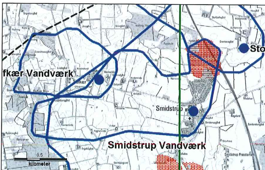
Figur 24. Indvindingsopland til Smidstrup Vandværk, med angivelse af indsatsområde med hensyn til nitrat og områder, hvor en indsats bør vægtes højt. Placering af geologisk profil (Figur 23), er angivet.
