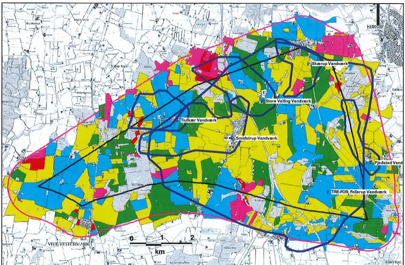
Figur 18. Estimeret kvælstofoverskud baseret på oplysninger fra GLR og gødningsregnskaber i 2001/2002. Fra/8/.
