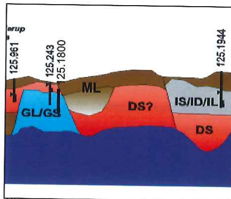
Figur 31 Geologisk principsnit gennem Pjedsted Vandværks kildeplads (syd-nord), se figur 32. (Legende henvises til figur 21.)
